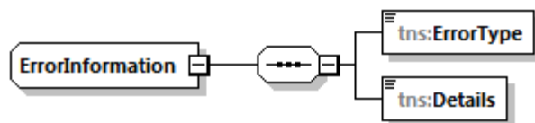
Bild 11: DmeErrorMessage – ErrorIdentifier:s struktur
