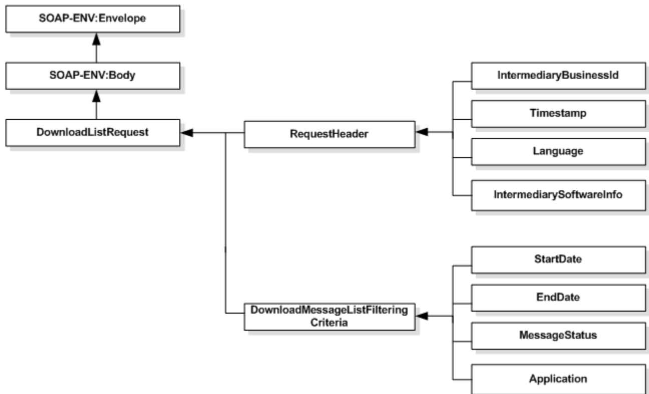
Bild 19: DownloadList, begäran med elementen StartDate och EndDate
