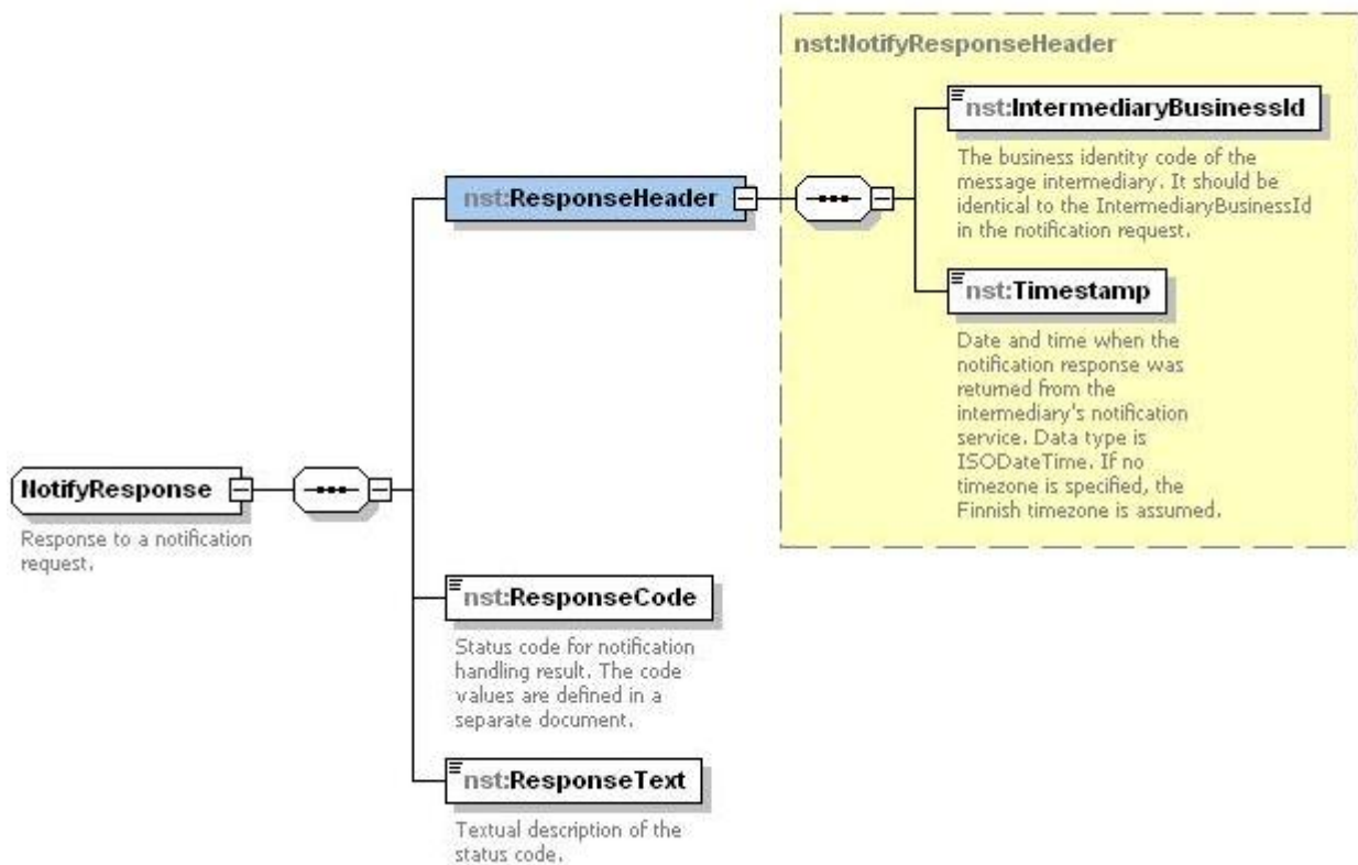
Bild 26: Beskrivning av NotifyResponse som skickas av kunden
