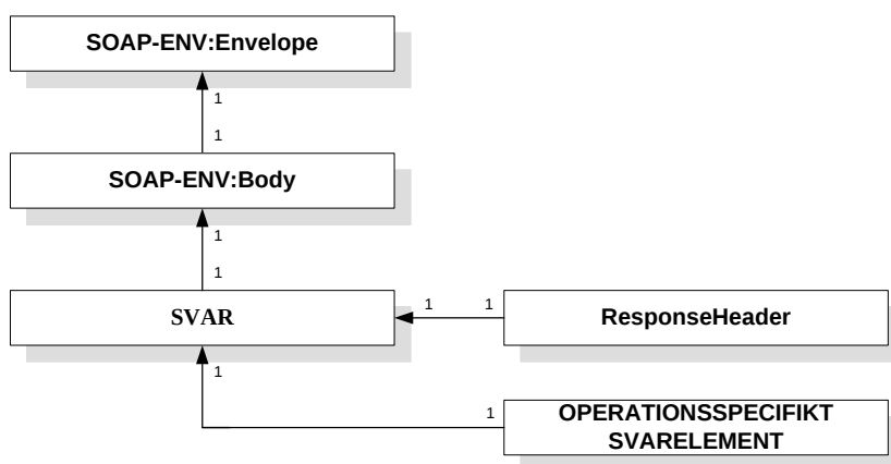
Bild 5: SOAP-svarsmeddelandets struktur på hög nivå
