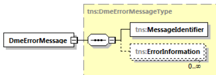
Bild 9: DmeErrorMessage:s struktur
