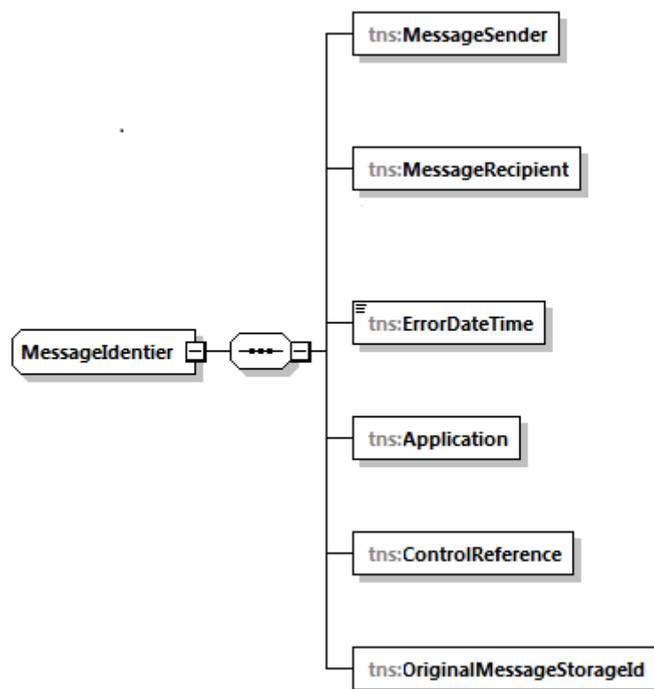
Bild 9: DmeErrorMessage:s struktur
