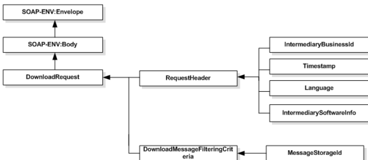
Bild 22: Download, begäran
