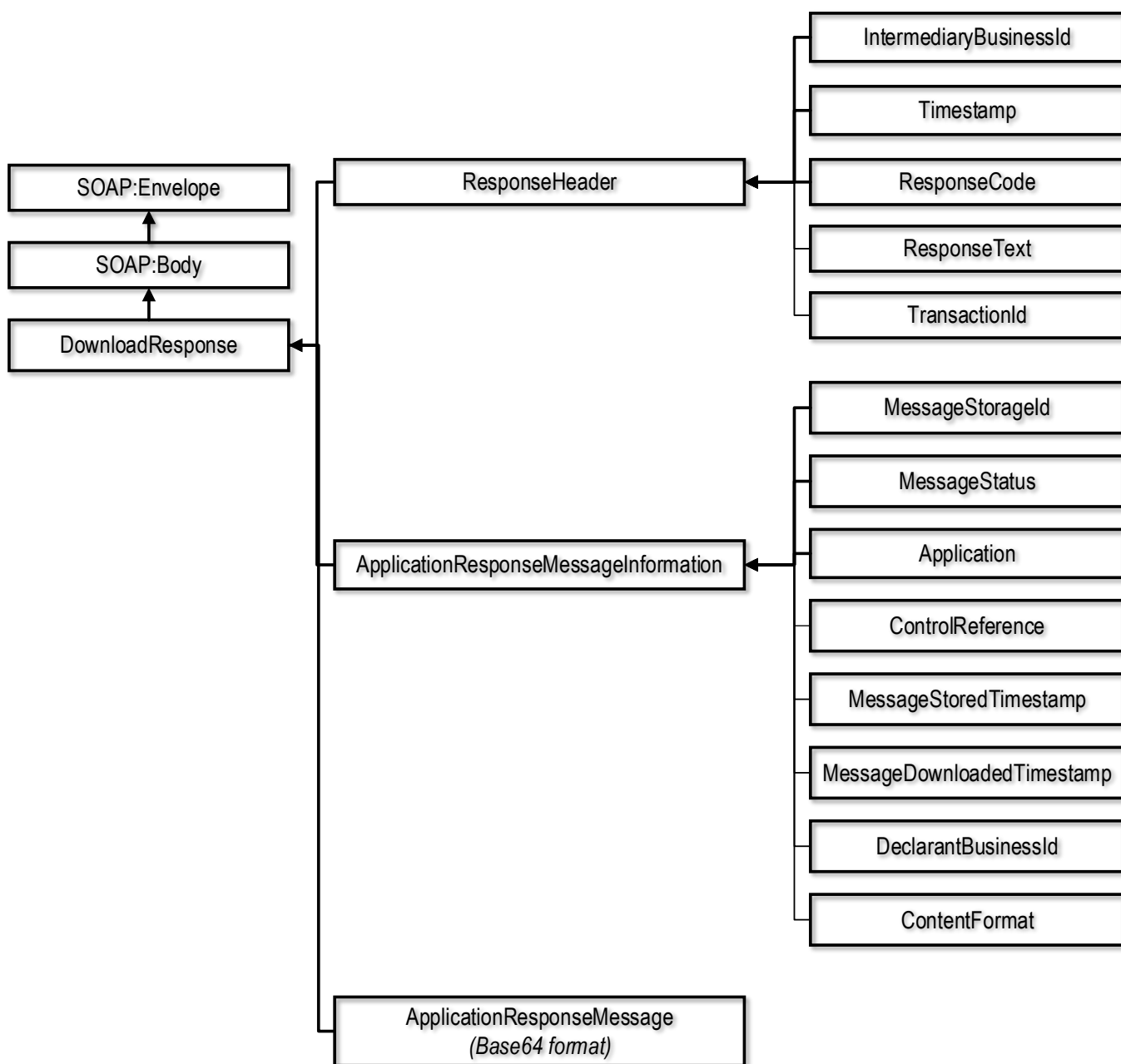
Bild 23: Download, svar
