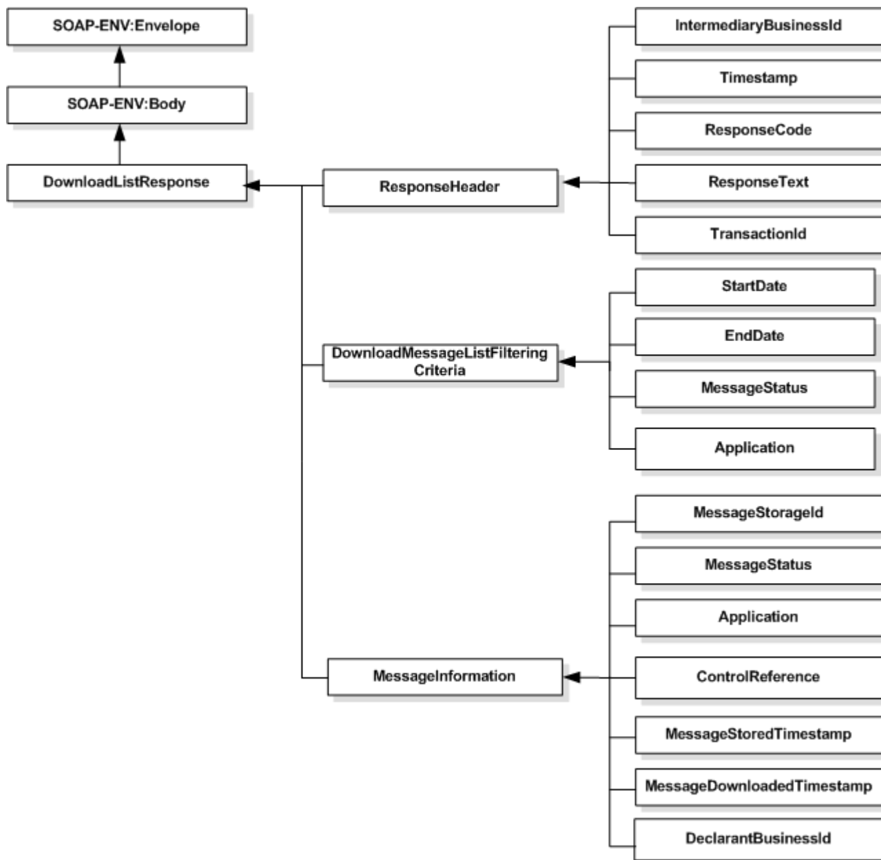
Bild 21: DownloadList, svar
